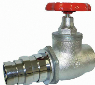
DV22-008 50A・65A×180° 差込式(マルチコネクト)
